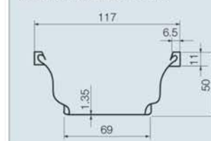
軒どい(117)断面図(位単位:mm)
